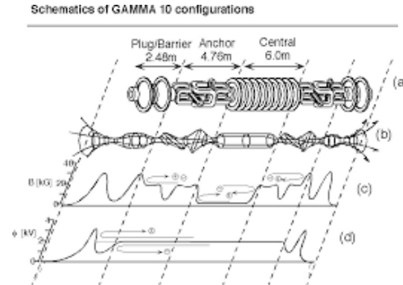
直線プラズマ実験
